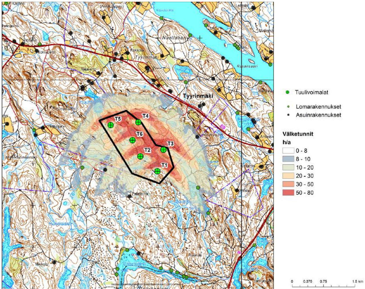
Kuva 9: Laskennallinen arvio tuulivoimapaiston aiheuttamasta todellisesta välketuntien määrästä.
