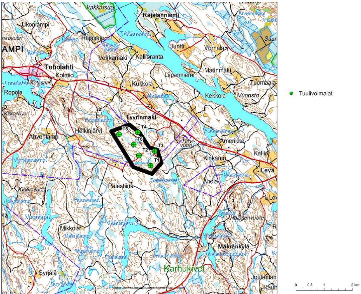
Kuva 2: Tuulivoimapuiston hankealue ja suunnitellut voimaloiden sijoituspaikat.
