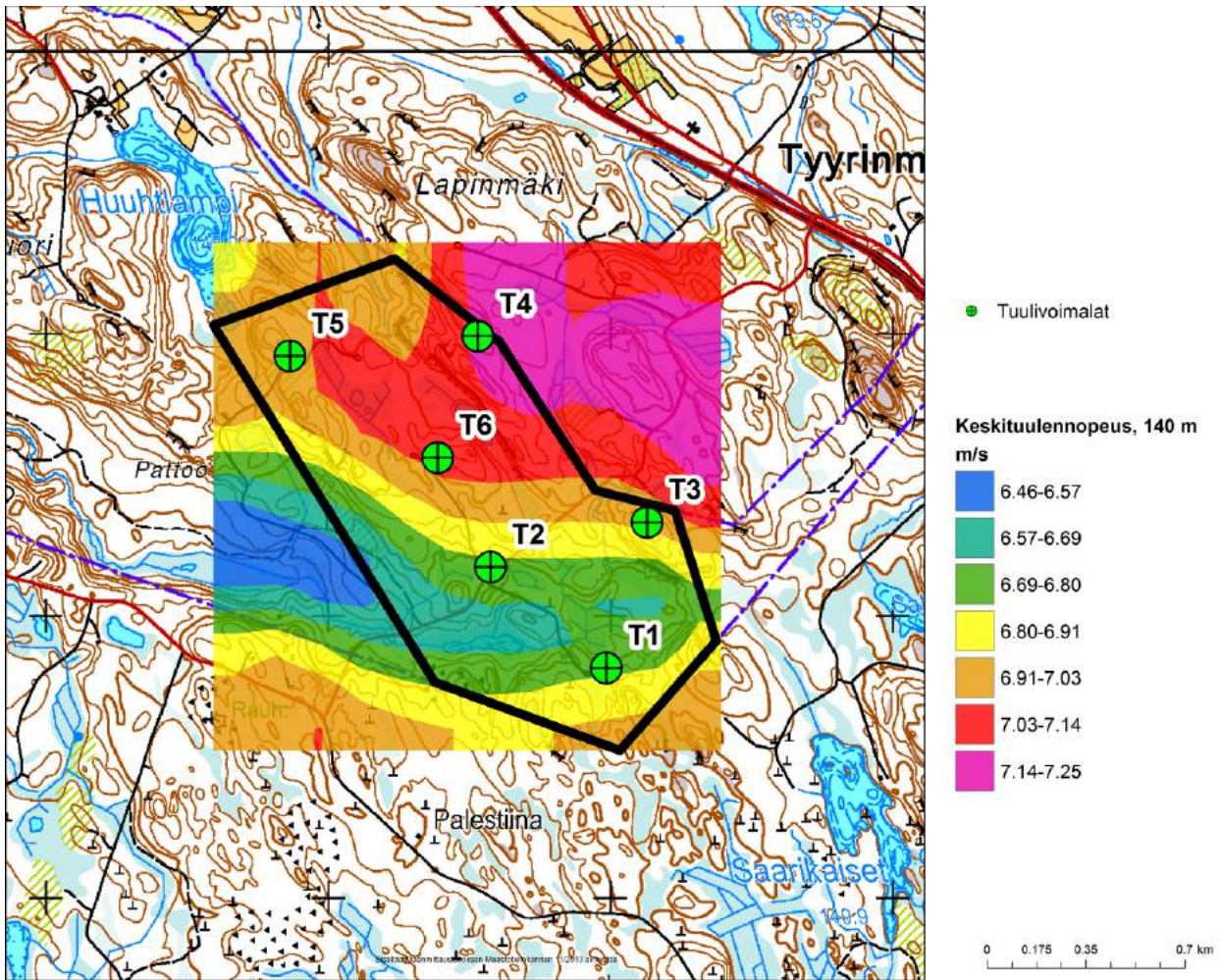
Kuva 21: Keskituulennopeudet tuulivoimapaiston alueella korkeudella 140 m.
