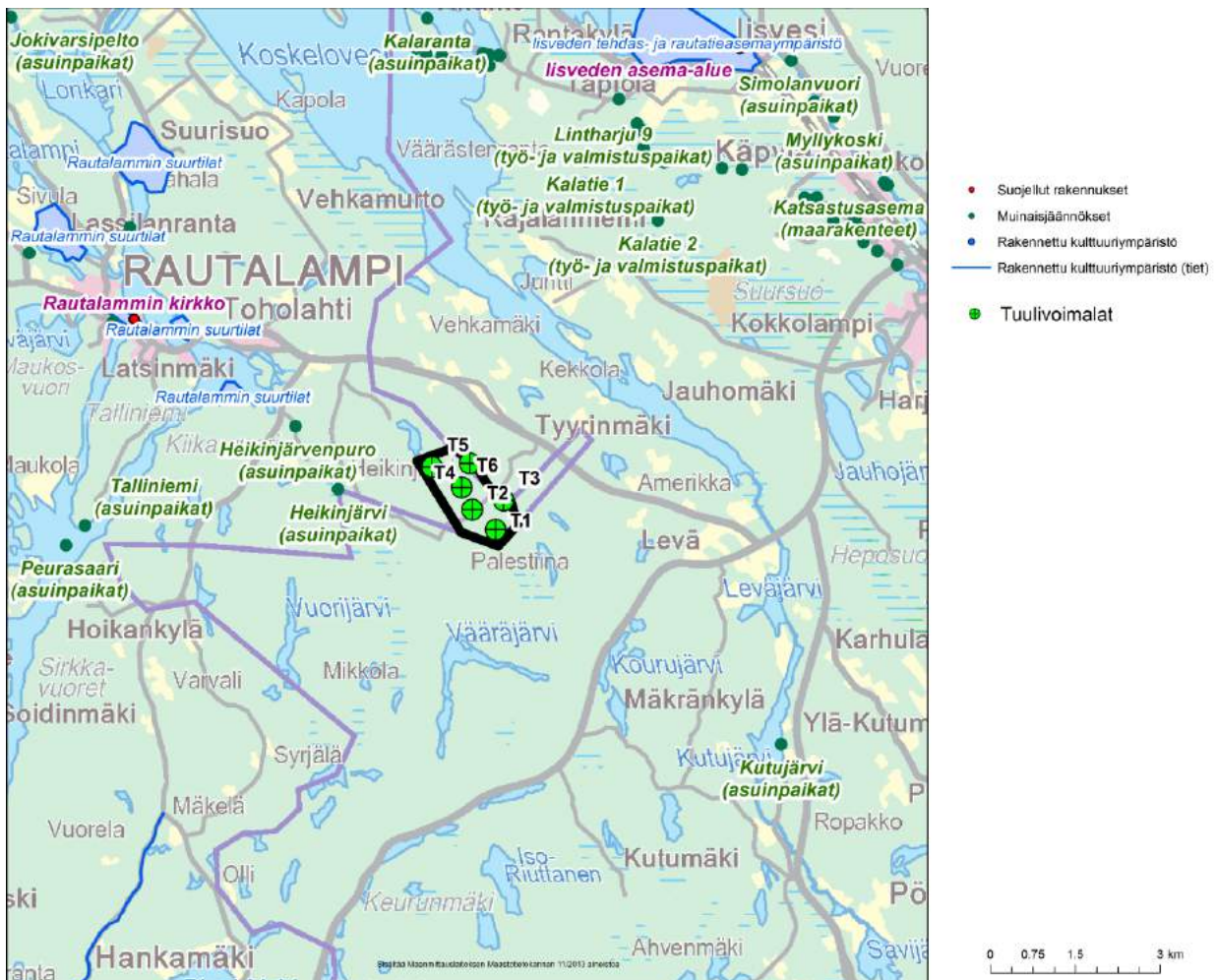
Kuva 19: Museoviraston paikkatietoaineiston sisältämät tuulivoimapuiston ympäristön suojellut kulttuuriympäristökohteet.
